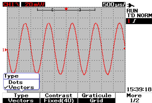
Abbildung 3-23 Anzeigetyp „Vectors“
