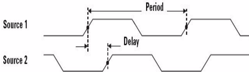
Abbildung 3-28 Phasenmessung
