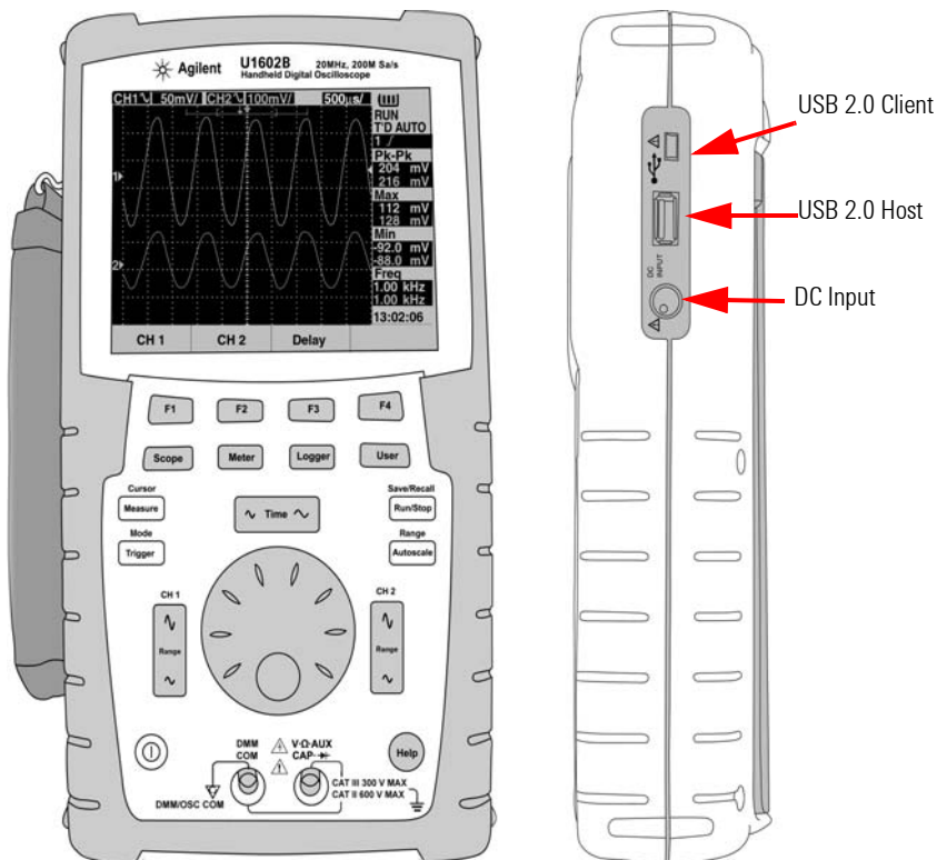
Abbildung 2-1 Bedienfeld des digitalen Handoszilloskops der U1600B-Serie
