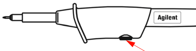
Abbildung 1-12 Trimmerwiderstand für das Ausgleichen der Messsonde
