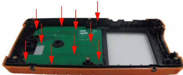
Abbildung 8-11 Entfernen Sie die zehn Schrauben von der vorderen Abdeckung
