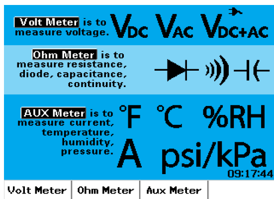
Abbildung 4-1 Multimeteranzeige
