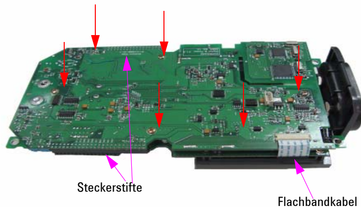
Abbildung 8-13 Entfernen Sie die sechs Schrauben und ziehen Sie das Flachbandkabel von der Leiterplatte ab
