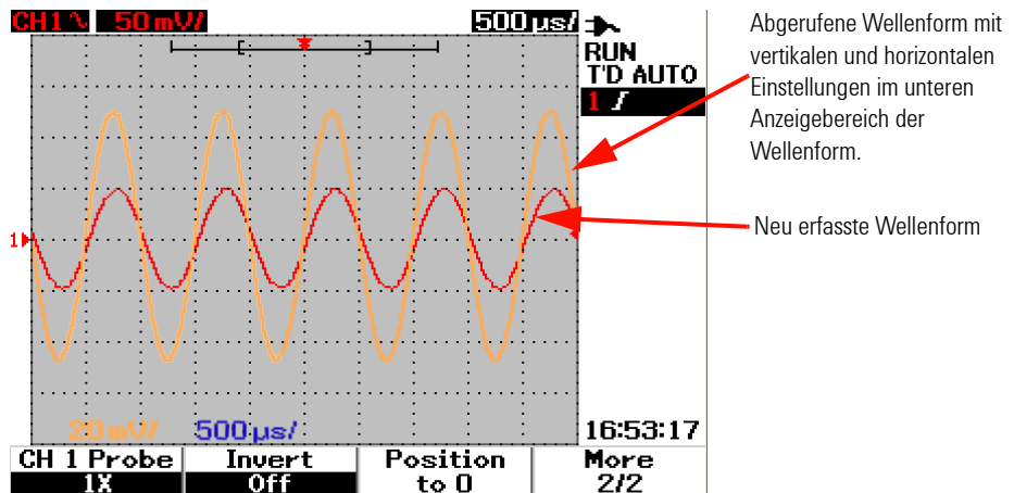
Abbildung 3-43 <Load> wird angezeigt, wenn eine Datei mit einer Wellenform unter „Waveform 1“ gespeichert wurde. Drücken Sie zum Aufrufen der Wellenform aus dem internen Speicher auf die Taste F1. Diese Funktion eignet sich für den Wellenformvergleich.
