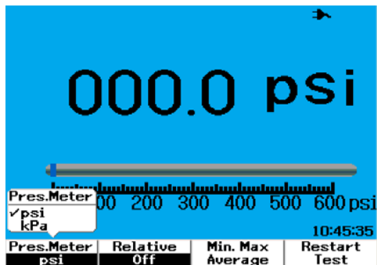
Abbildung 4-11 Druckmessung
