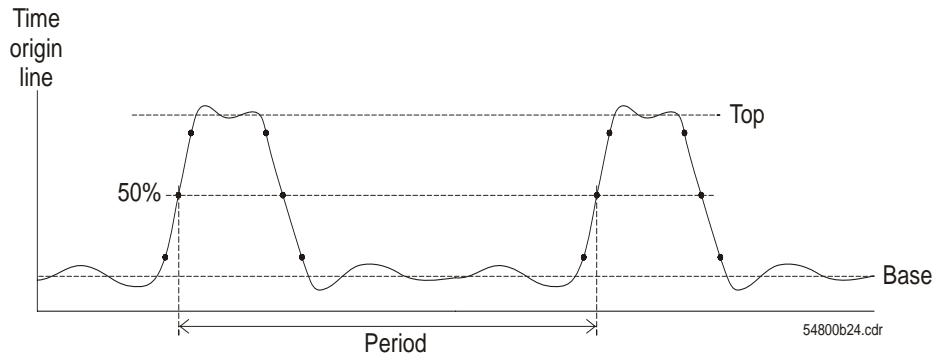
Abbildung 3-26 Zeitraummessung
