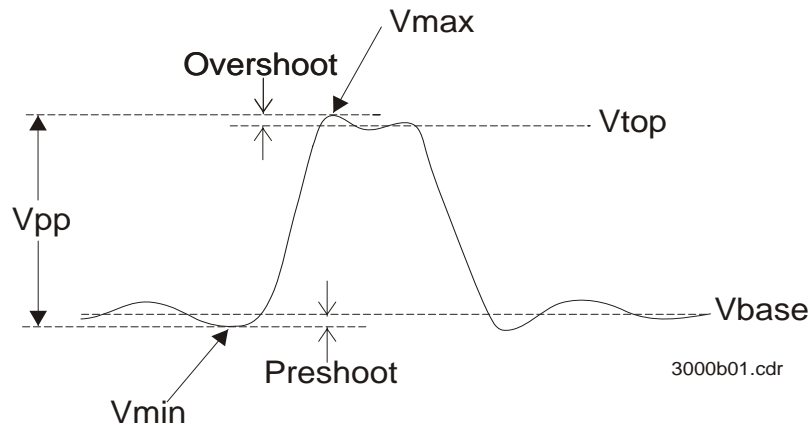
Abbildung 3-27 Spannungsmessung
