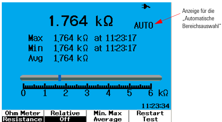
Abbildung 4-16 Modus „Automatische Bereichsauswahl“
