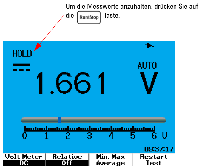
Abbildung 4-2 DC-Messanzeige
