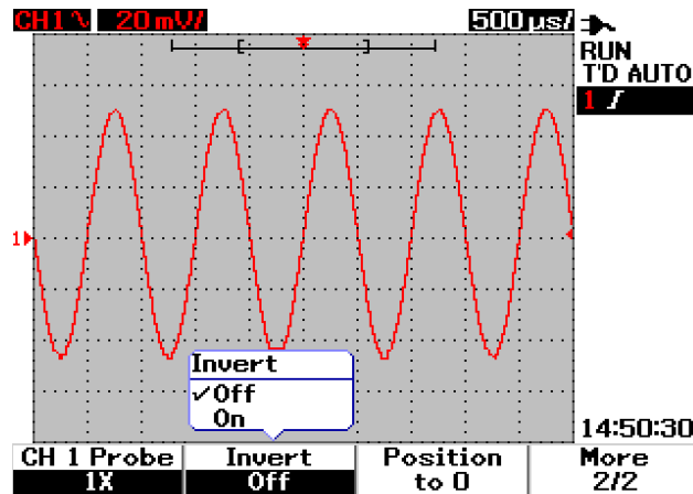
Abbildung 3-10 Die Wellenform vor der Umkehrung.
